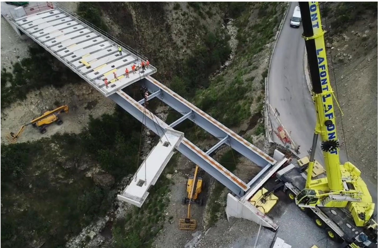
Pose des dalles préfabriquées - Cozzi-Colas - 2022
