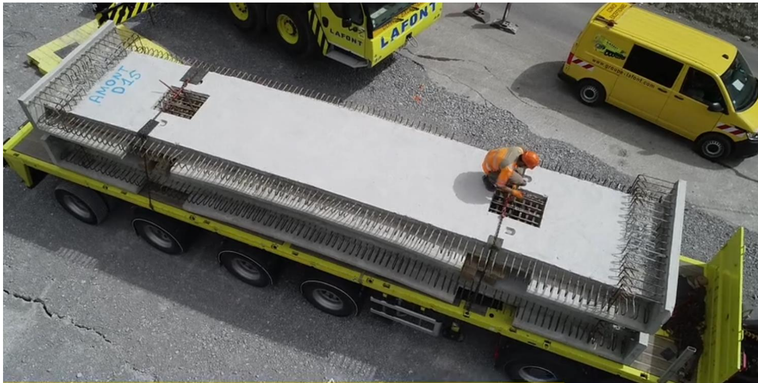
Dalles préfabriquées - Cozzi-Colas - 2022
